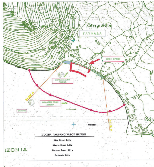
ΑΠΟΠΛΑΙΣΜΑ ΠΙΝΑΚΙΔΑΣ ΓΥΤ φ. 4218.2 - Κλίμακα 1:5000 ΔΙΑΓΡΑΜΜΑ ΧΕΡΣΙΑΣ & ΘΑΛΑΣΣΙΑΣ ΣΤΟΝ ΛΙΜΕΝΑ ΓΛΥΦΑΔΑΣ
