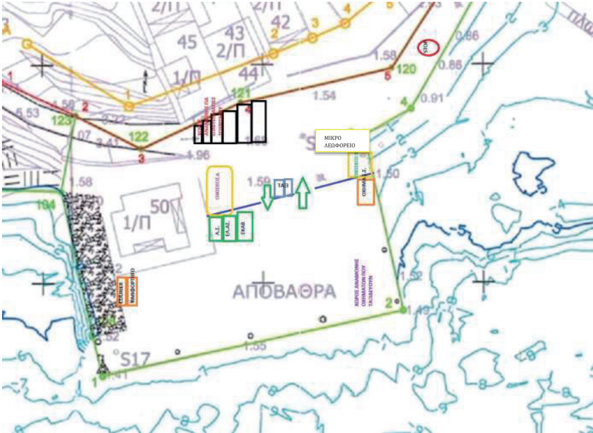
ΤΟΠΟΓΡΑΦΙΚΟ ΔΙΑΓΡΑΜΜΑ 01
