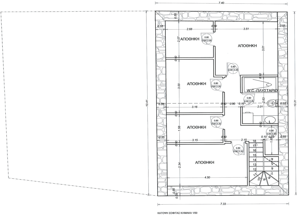
ΚΑΤΟΨΗ ΣΟΦΙΤΑΣ ΚΛΙΜΑΚΑ 1/50
