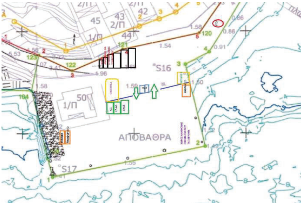
ΤΟΠΟΓΡΑΦΙΚΟ ΔΙΑΓΡΑΜΜΑ 01
