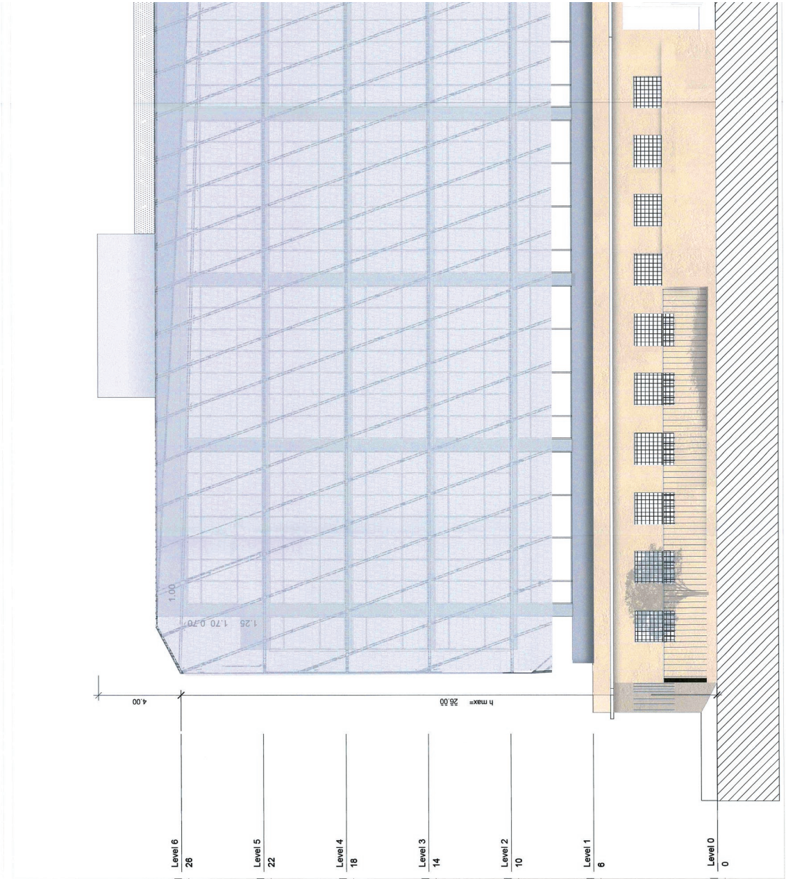
2 Βορειοδυτική Όψη 1 : 100
