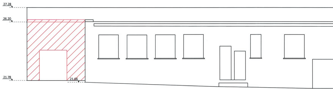
ΟΨΗ Ε3
